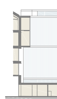
DWARSSNEDE PATIO
