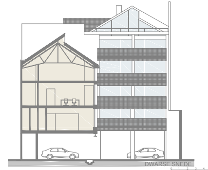
DWARSSNEDE
