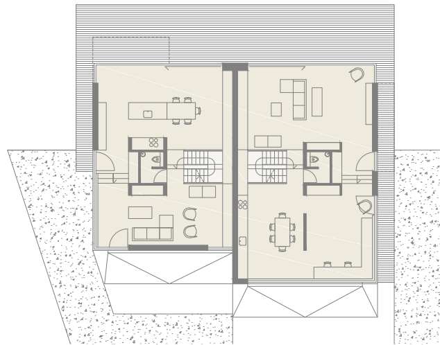
VERDIEPING +1
