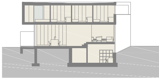
DWARSSNEDE
