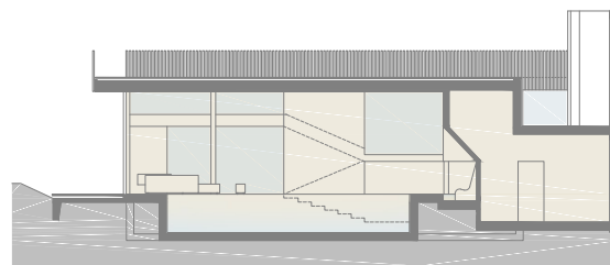
LANGSSNEDE
