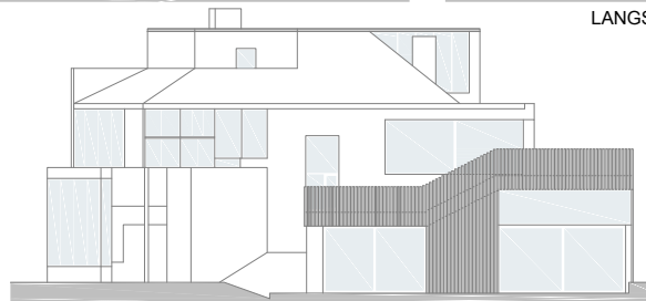
ZUIDGEVEL
