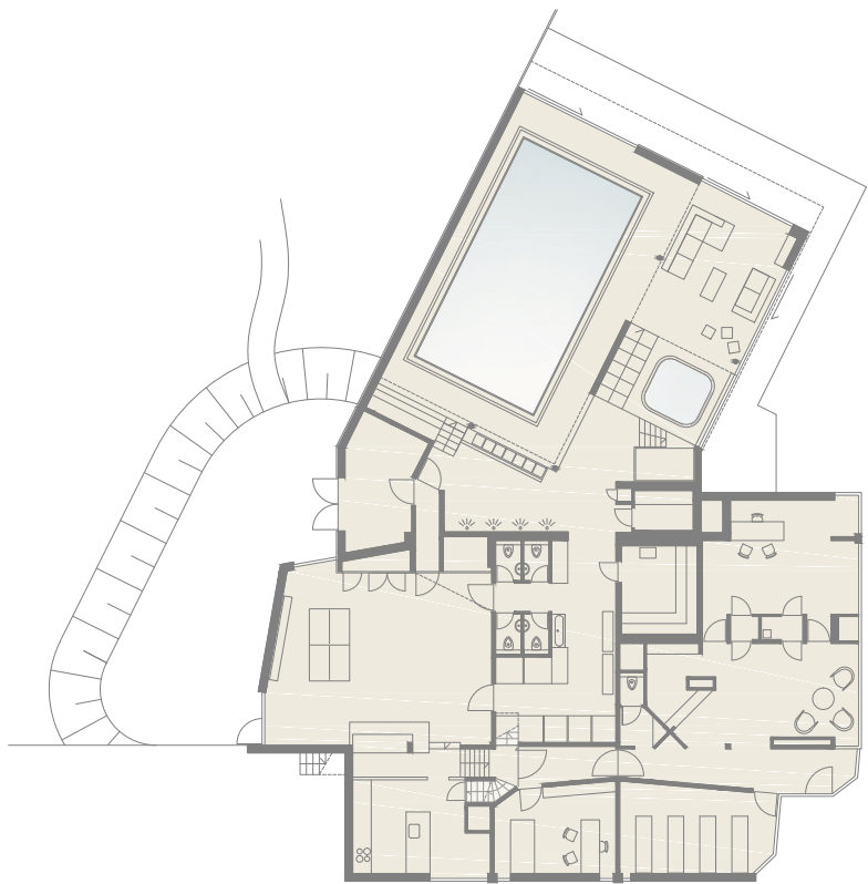
VERDIEPING 0
