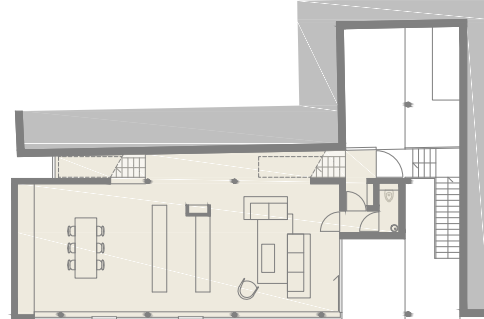
VERDIEPING +1
