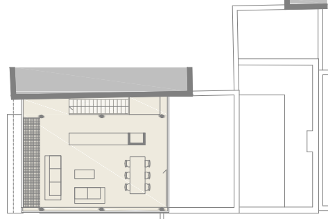
VERDIEPING +4
