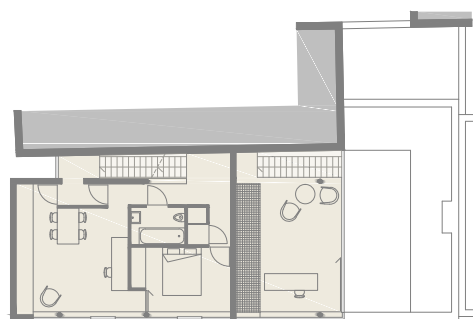
VERDIEPING +3
