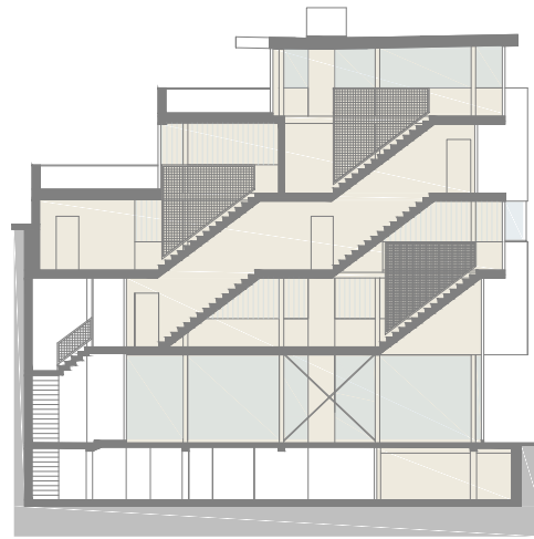
LANGSSNEDE
