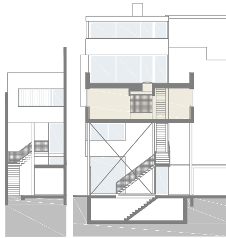
DWARSSNEDE
