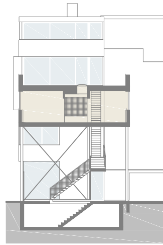
DWARSSNEDE
