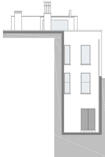
WESTGEVEL
