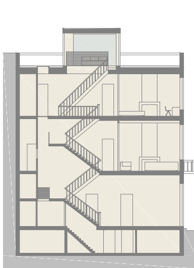
LANGSSNEDE
