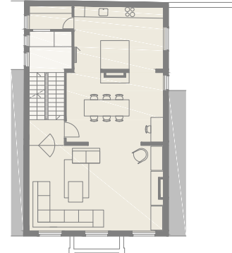
VERDIEPING +1
