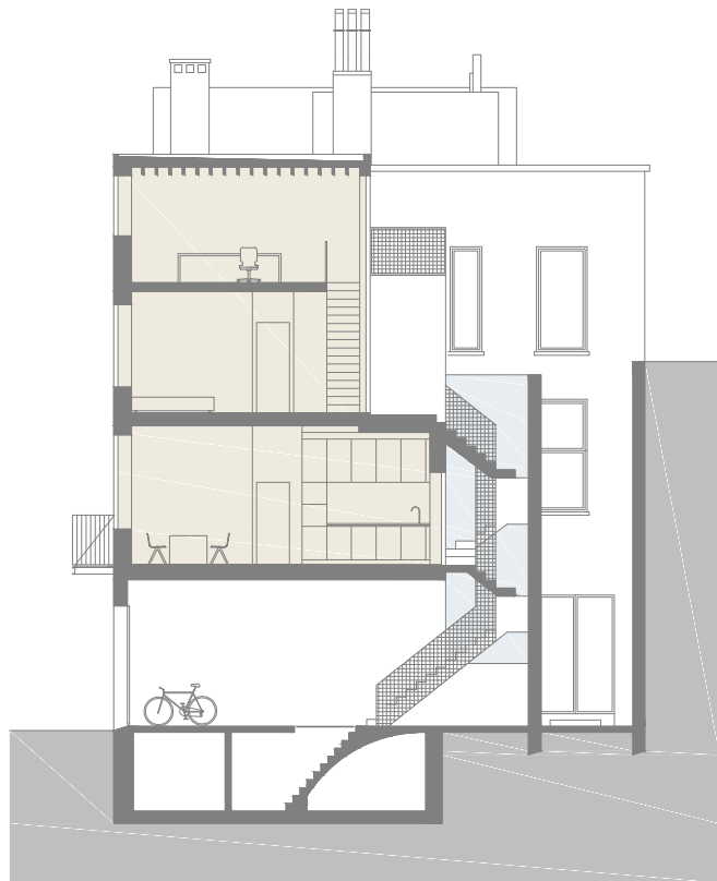
LANGSSNEDE
