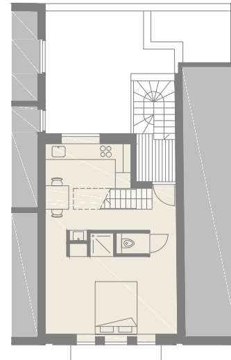
VERDIEPING +2
