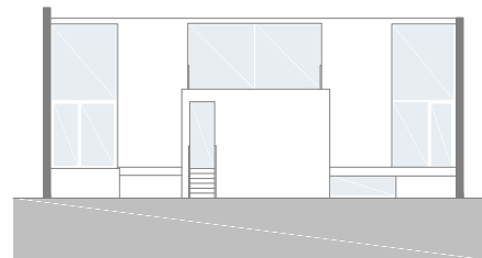
OOSTGEVEL
