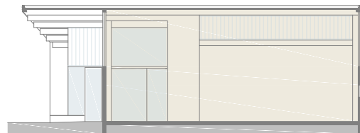
DWARSSNEDE
