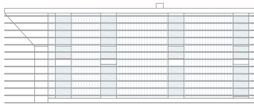
OOSTEGEVEL
