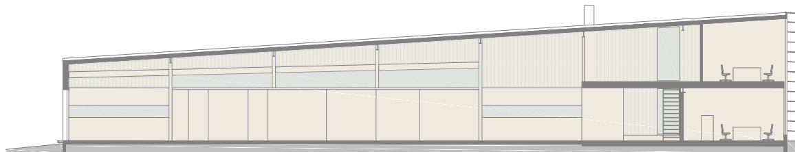
LANGSSNEDE
