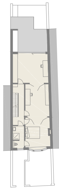
VERDIEPING +2
